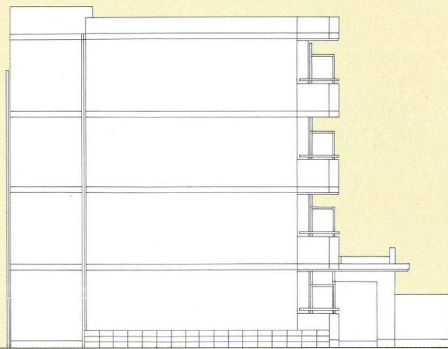
北側立面図
