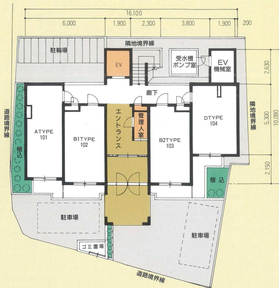
配置図・1 F平面図
